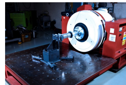
진동 시험
