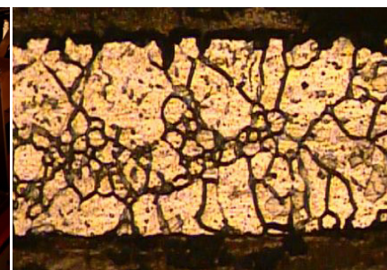
소재부식 시험
