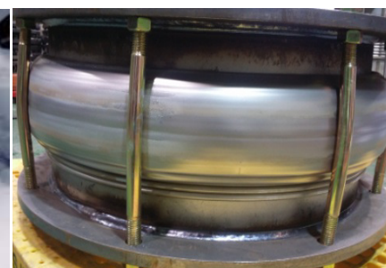
파열시험
